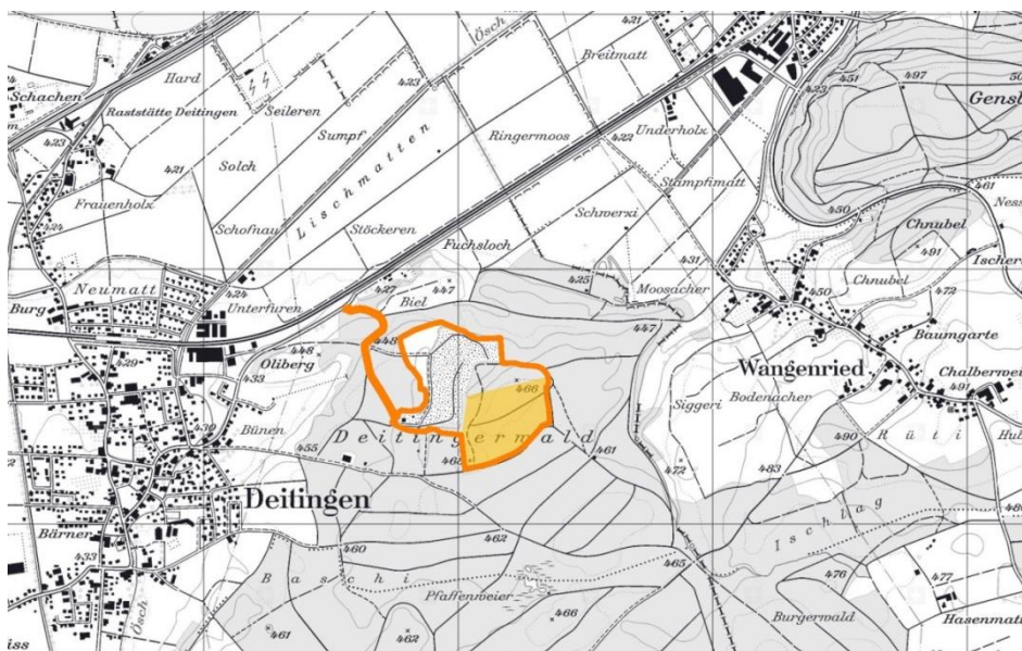
Abbildung 1: Übersicht Kiesgrube Mühlerain, orange: Gestaltungsplanperimeter, gelbe Fläche: Erweiterung Kiesabbau, Festsetzung gemäss kantonalem Richtplan
